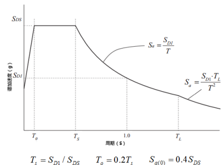
图 1 ASCE7-10 设计反应谱
